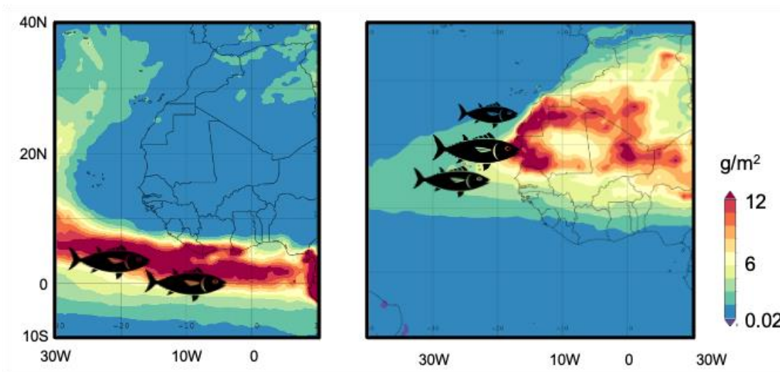
Ubicación de los caladeros de pesca del atún listado en invierno (izquierda) y en verano (derecha), situados en las zonas de mayores tasas de deposición de polvo desértico. Imagen extraída del estudio
